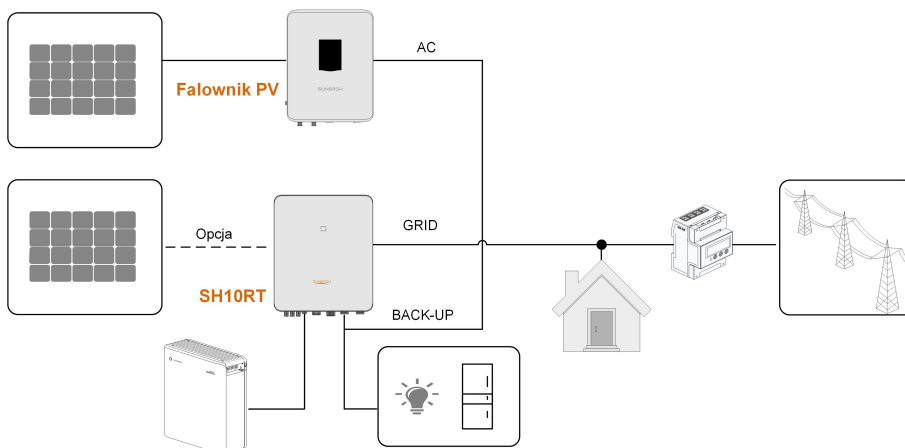
Rys. 2-6 Złącze off-grid do doposażania istniejącej instalacji PV
