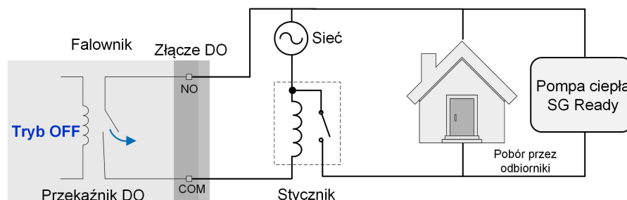
Rys. 8-23 Działanie DO w trybie przełączania
