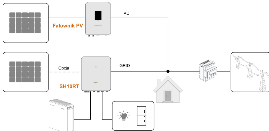
Rys. 2-5 Złącze on-grid do doposażania istniejącej instalacji PV
