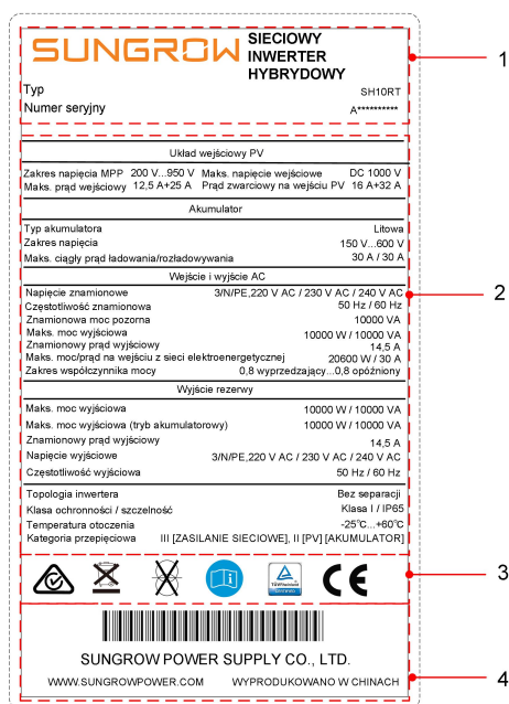
Rys. 4-1 Tabliczka znamionowa falownika
