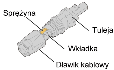
Rys. 6-3 Elementy złącza SUNCLIX
