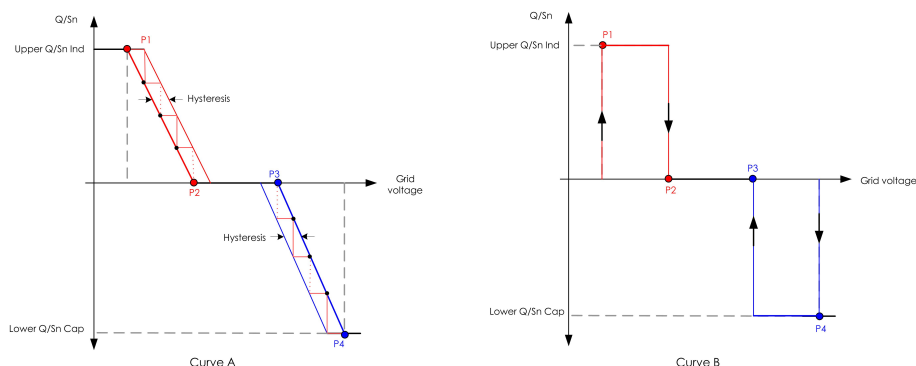
Rys. 8-4 Krzywa Q(U)
