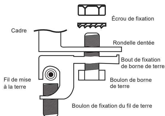
Figure 12 Méthode d'Installation
