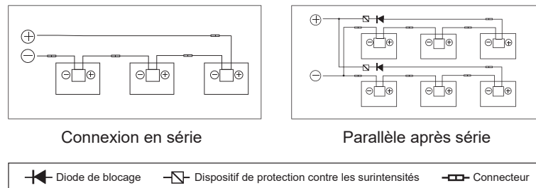
Figure 10 Schéma de connexion en série et en parallèle
