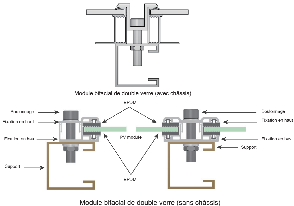
Figure 8 Installation du module bifacial par des outillages de fixation
