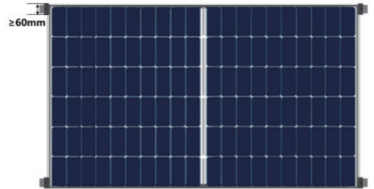
Les outillages de fixation sont montés aux coins du cadre court. (La longueur de la pièce de fixation \geq 60\text{mm} , le chevauchement entre la pièce de fixation et le cadre \geq 9\text{mm} )
