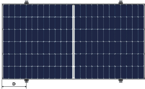
Installation avec des outillages de fixation au côté long du module encadré (Support transversal perpendiculaire aux côtés longs) (longueur de pièce \geq 50\text{mm} )
