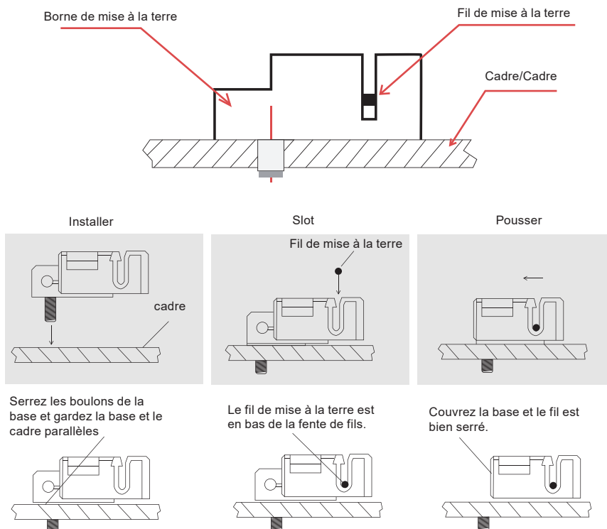
Figure 11 Installation de la borne de mise à la terre
