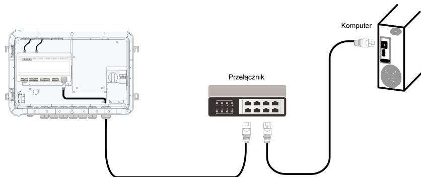
Rys. 5-2 Połączenie z systemem zaplecza PV
