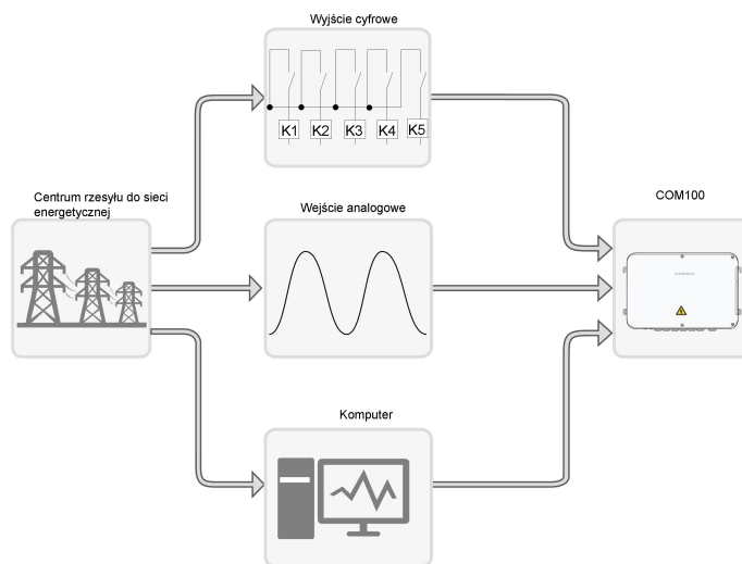
Rys. 7-1 Ogólna rama funkcji sterowania mocą
