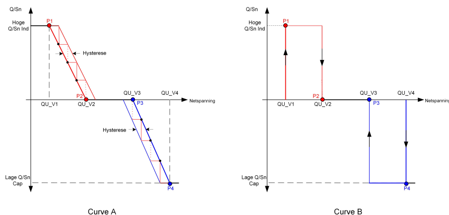
Afbeelding 8-5 Q(U) curve
